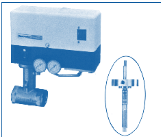
Рис. 13 Сильфонный ВАРИПАК (на выноске - сильфонная сборка)
