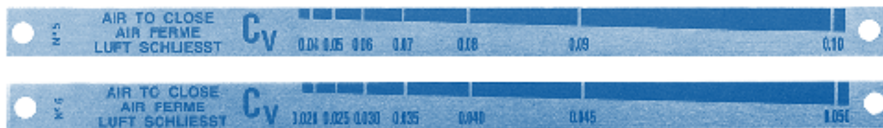
Рис. 5 Шкала C_v для затворов №№ 5 и 6
