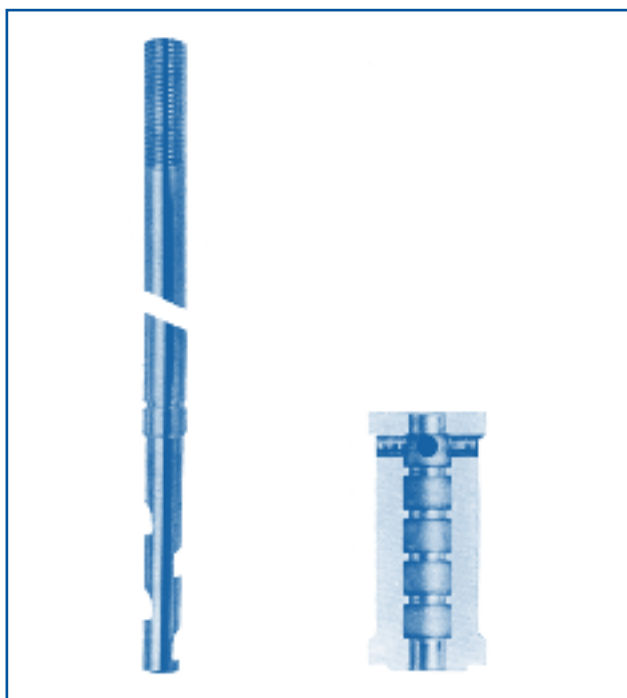
Рис. 11 Узел затвора
