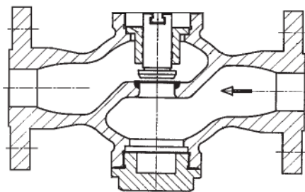
AT/S1/D (DN20-25-32-40-50)
