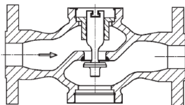
AT/S1/R (DN20-25-32-40-50)
