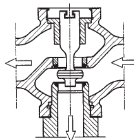
AT/3V/DV
