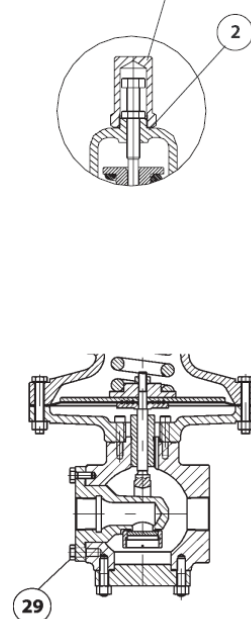
Исполнение с герметичной крышкой
