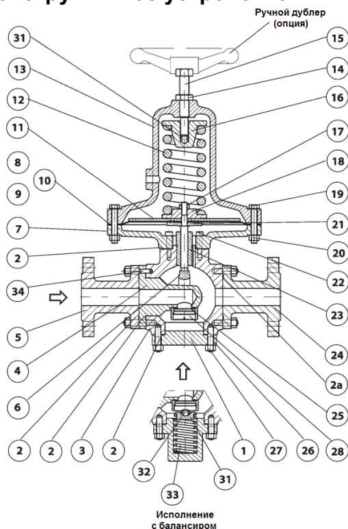
Фланцевое присоединение
