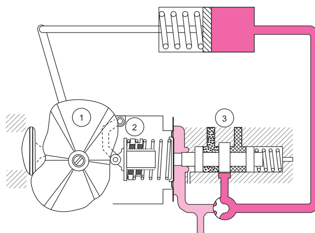
Позиционер обратного действия (только 4700Р)
