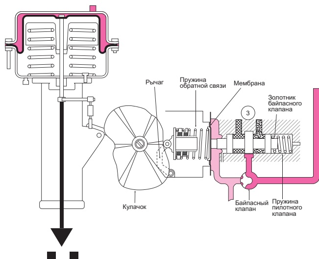
Рис. 2. Линейный привод
