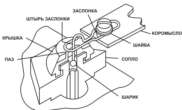
Рис. 1. Сборка сопла
