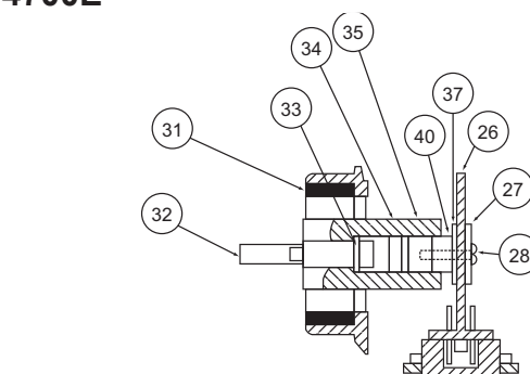
Поворотный привод
