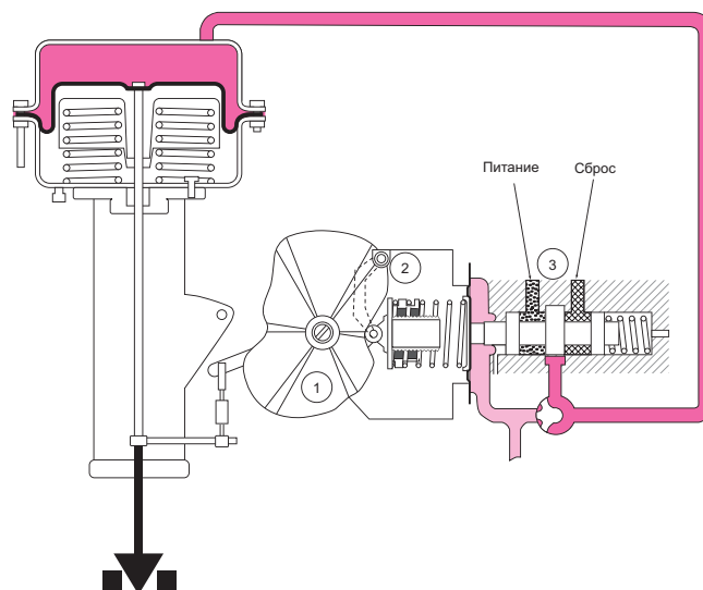
Рис. 2. Линейный привод
