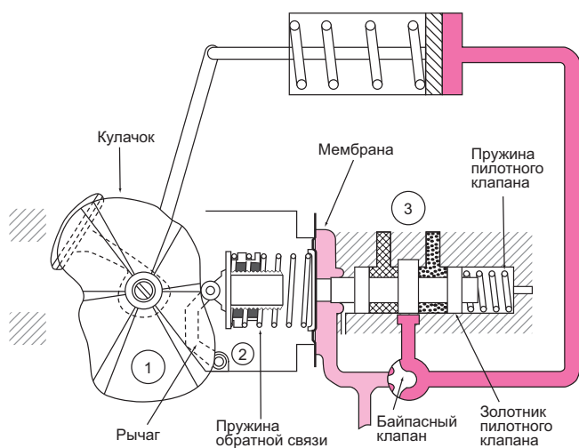
Рис. 1 Поворотный привод
